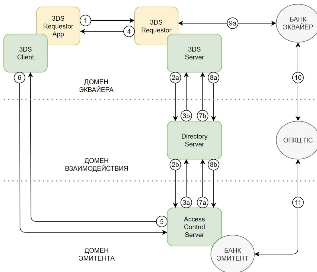
Рисунок 1 – Схема взаимодействия участников протокола 3D Secure 2.0
